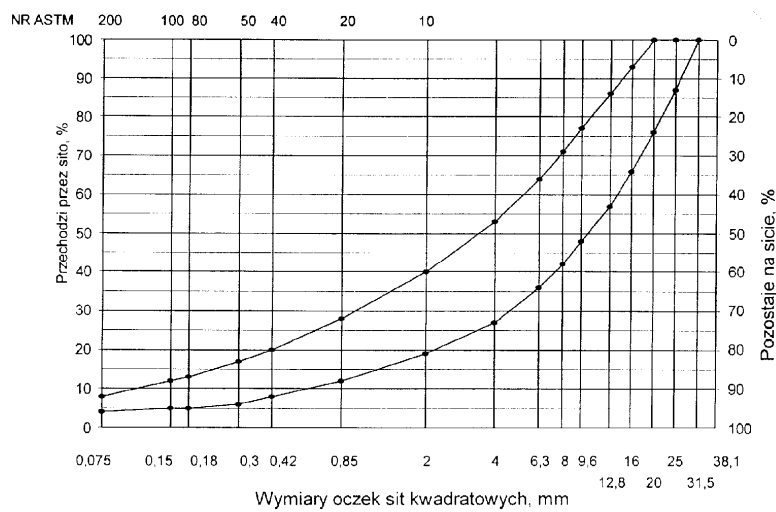
ys. 2. Krzywe graniczne uziarnienia mieszanki mineralnej BA od 0 do 25mm do podbudowy nawierzchni drogi o obciążeniu ruchem KR1 lub KR 2
